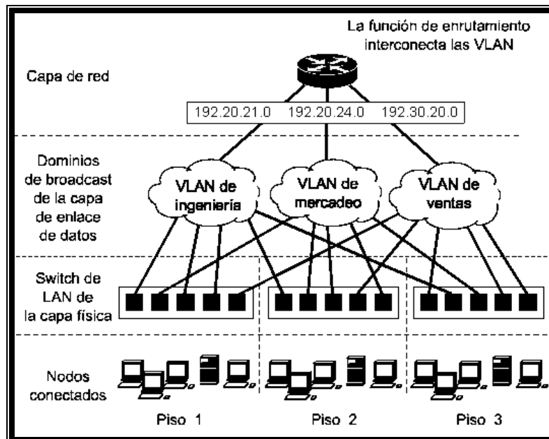
Figura 1.15.- VLAN de puerto central
