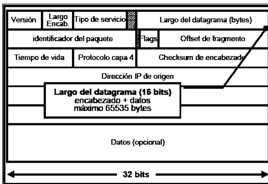
Figura 3.21.- Estructura de un datagrama IP v4, largo del datagrama.
