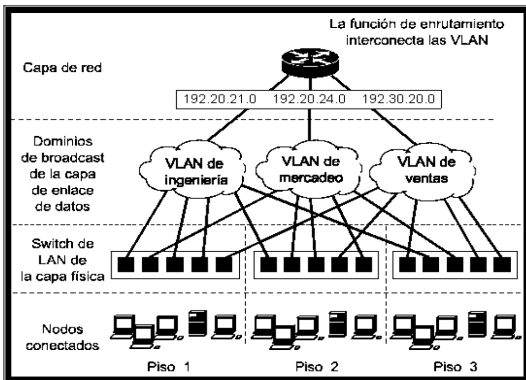
Figura 2.- VLAN de puerto central
