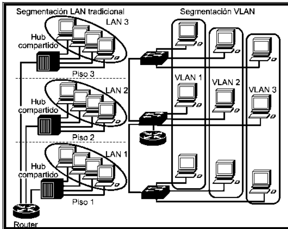
Figura 1.13.- Las VLAN y los límites físicos
