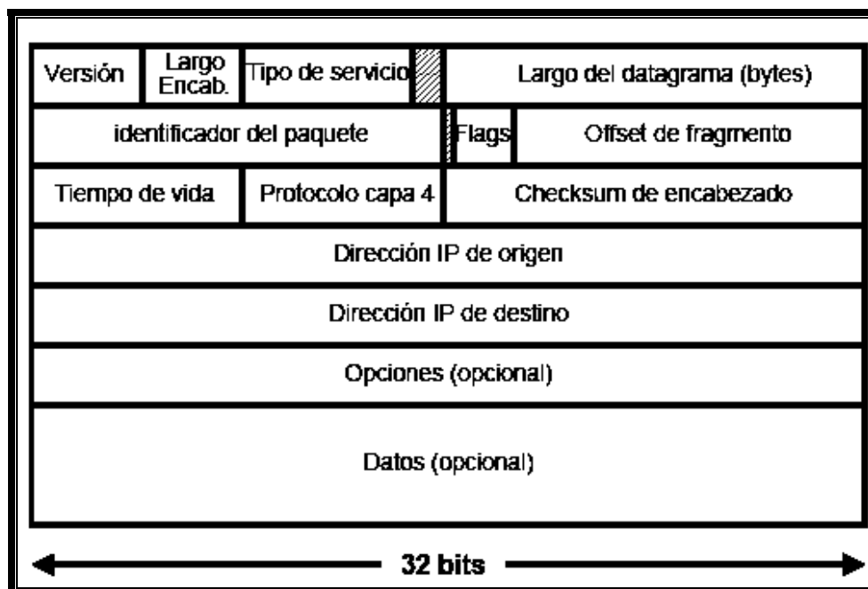
Figura 3.18.- Estructura de un datagrama IP v4, campo versión.
