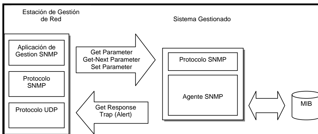
Figura 2.1.- Elementos de SNMP.
