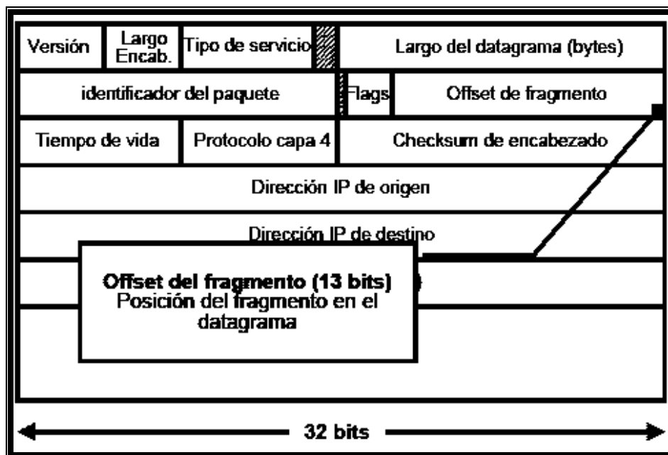
Figura 3.24.- Estructura de un datagrama IP v4, offset del fragmento.
