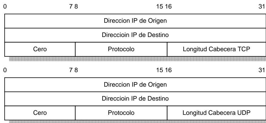
Figura 3.18.- Pseudo-cabecera TCP, UDP
