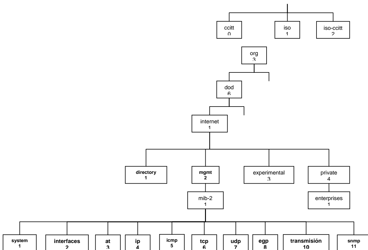
Figura 2.3.- Estructura de la MIB
