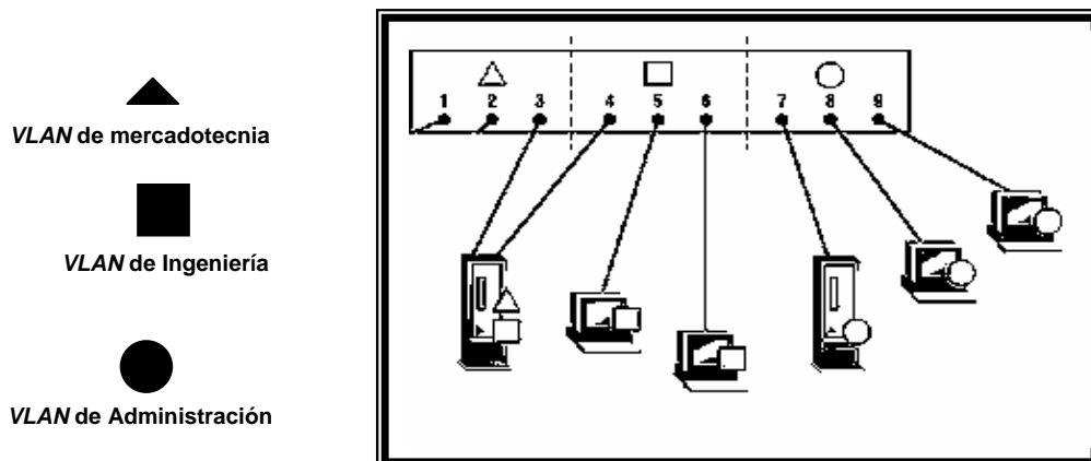
Fig.3.10 Conexión de un servidor de monitoreo a la infraestructura de VLAN.
