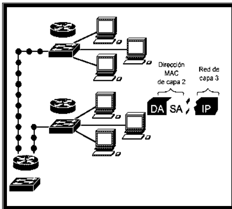
Figura 3.14.- Direcciones a tomar en cuenta en el monitoreo de VLAN's, destaca en importancia la dirección de capa tres de acuerdo al estándar RFC 3069 y RFC 2643.
