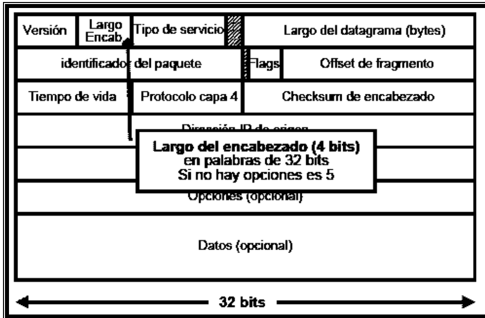
Figura 3.19.- Estructura de un datagrama IP v4, largo del encabezado.
