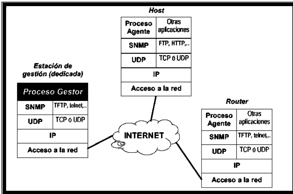
Figura 7.- Modelo de configuración estación Gestora y sistemas Gestionados.
