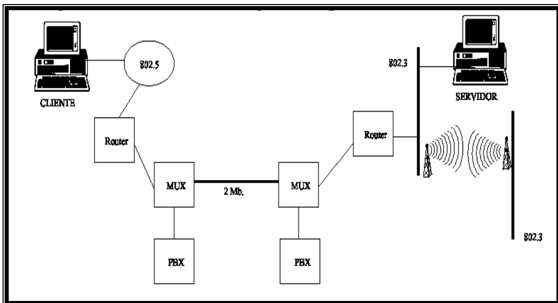
Figura 1.1.- Gestión de Fallos en una red.
