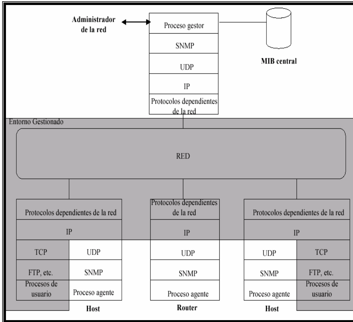
Figura 3.4.- Modelo de configuración estación SNMP Gestor y Agente.
