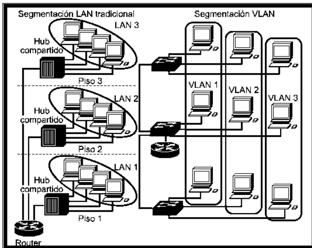
Figura 1.- Las VLAN y los límites físicos
