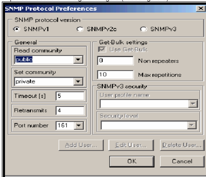
Figura 5.- Opciones de configuración para SNMP en MIB BROWSER
