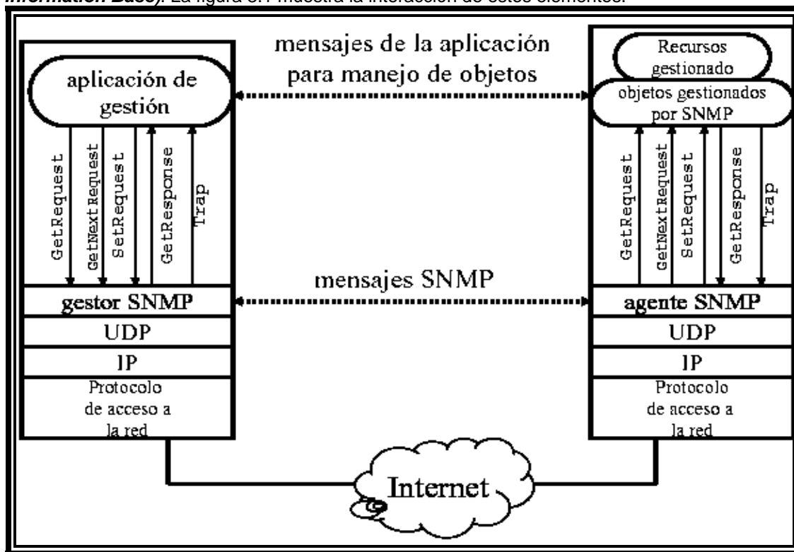
Figura 3.1. Elementos dentro de un entorno gestionado por SNMP.
