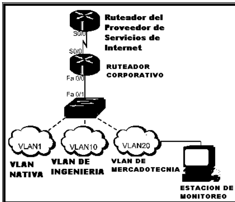
Figura 4.1.- Topología de Prueba para la Herramienta de Gestión de Redes Virtuales.
