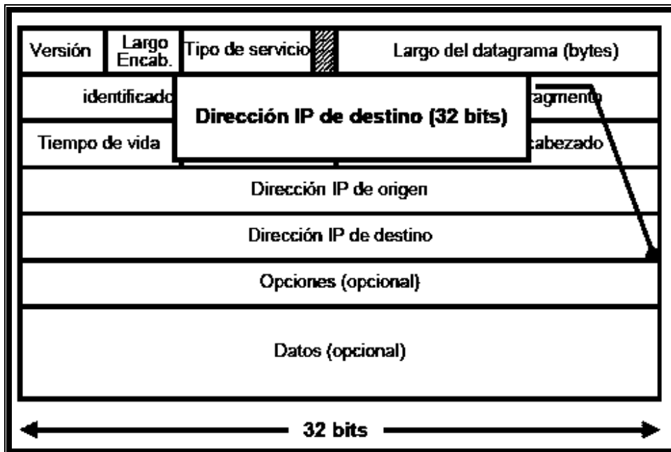
Figura 3.30.- Estructura de un datagrama IP v4, direcciones IP Destino.
