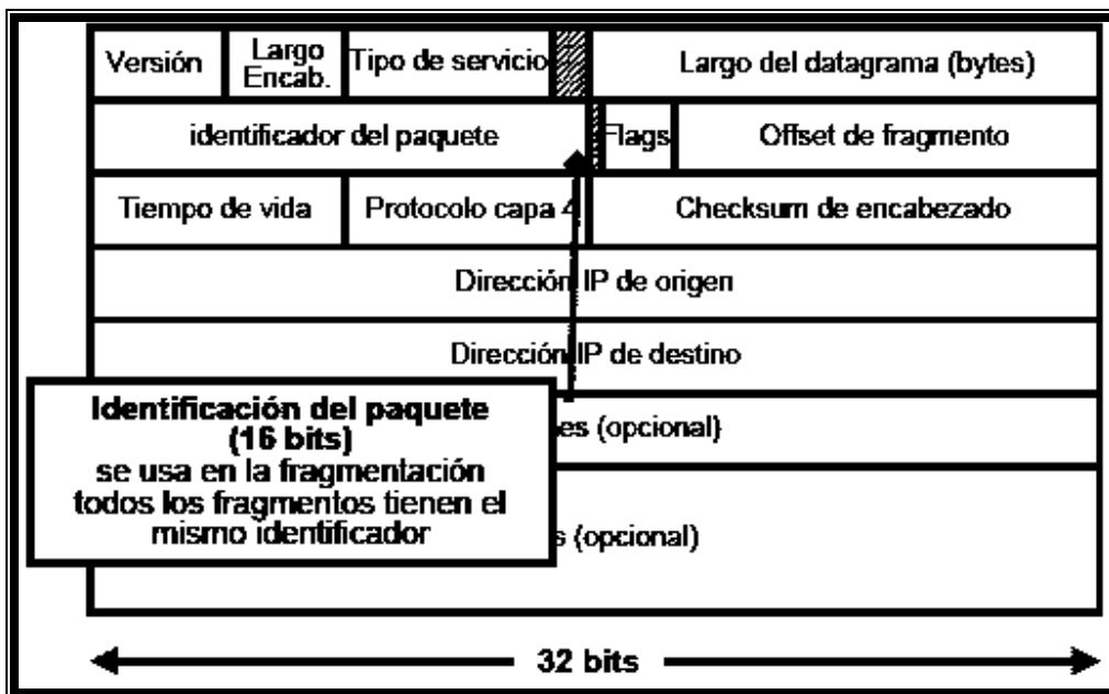
Figura 3.22- Estructura de un datagrama IP v4, identificación del paquete.
