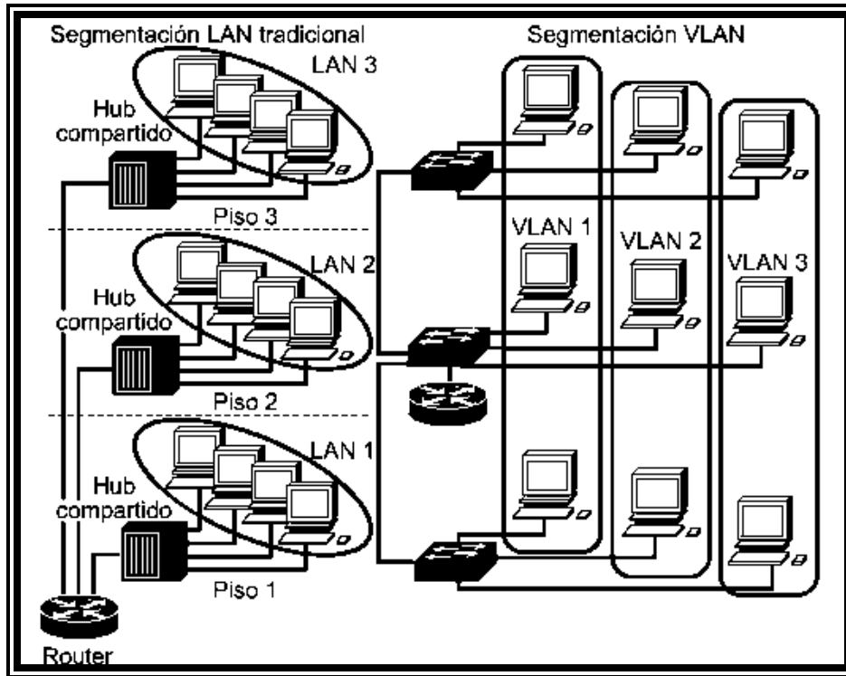
Figura 3.9.- Segmentación en una LAN tradicional y segmentación VLAN.
