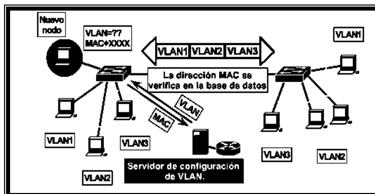
Figura 1.17.- VLAN dinámicas
