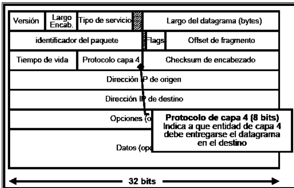
Figura 3.26.- Estructura de un datagrama IP v4, Protocolo de capa 4.
