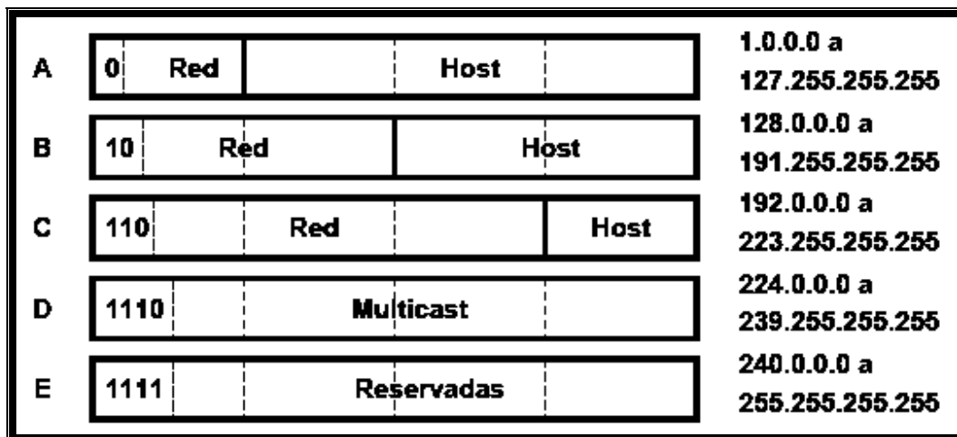
Figura 3.28.- Formato de Direcciones IP.
