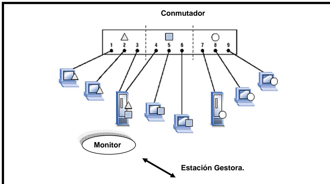
Figura 4.19.- Localización del programa de monitorización en las VLAN's
