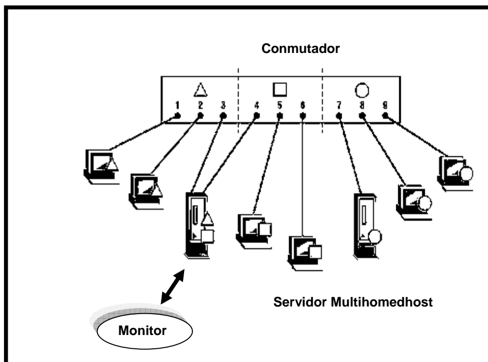
Figura 3.11.- Localización del programa de monitorización en las VLAN's
