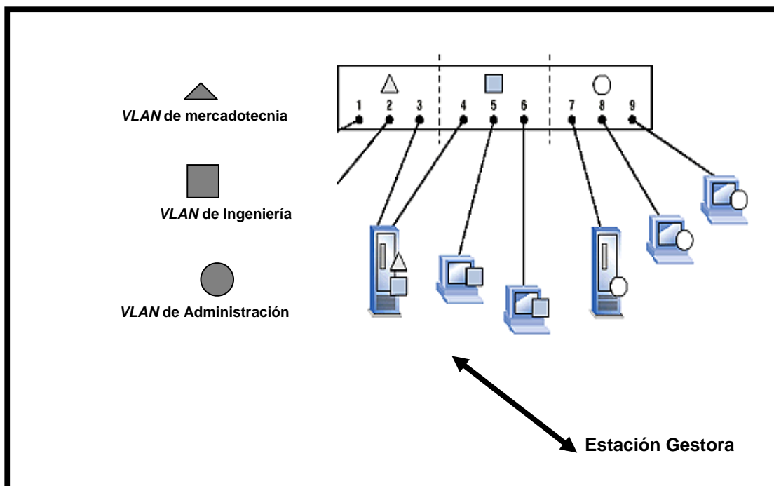
Figura 4.18.- Conexión de la estación gestora para el monitoreo de la VLAN.
