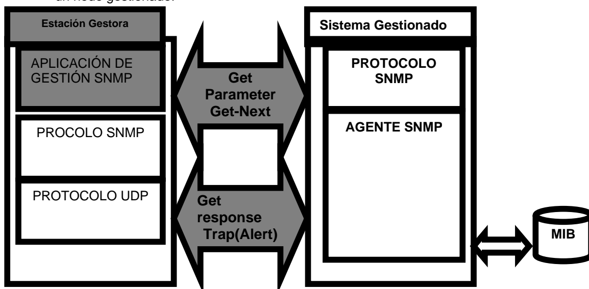
Figura 3.2.- Componentes del programa de configuración para redes virtuales. La parte sombreada representa lo que implementa el programa de configuración.
