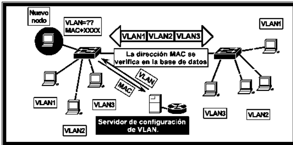
Figura 4.- VLAN dinámicas
