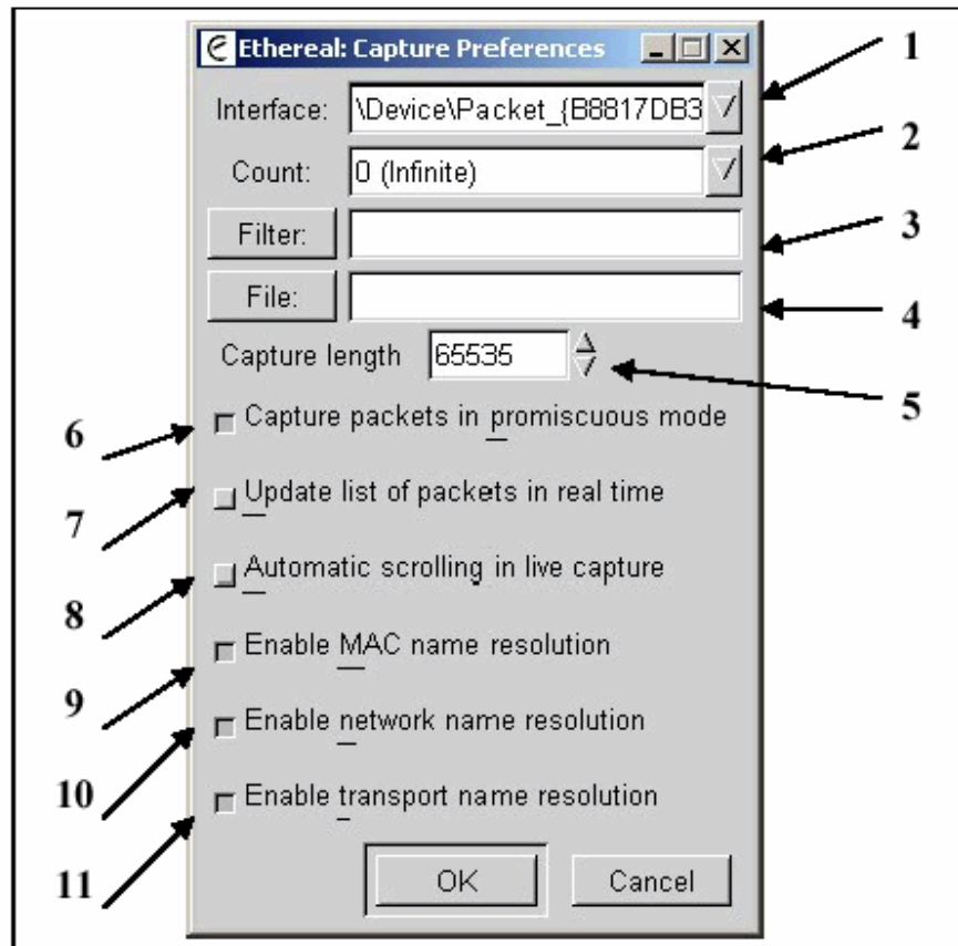
Figura 9.- Ventana de preferencias de Captura.
