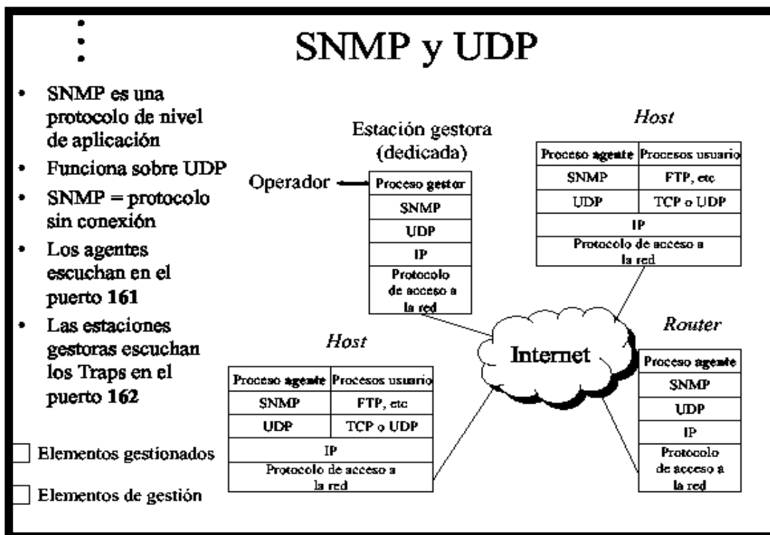
Figura 4.2.- Modelo de configuración estación Gestora y sistemas Gestionados.
