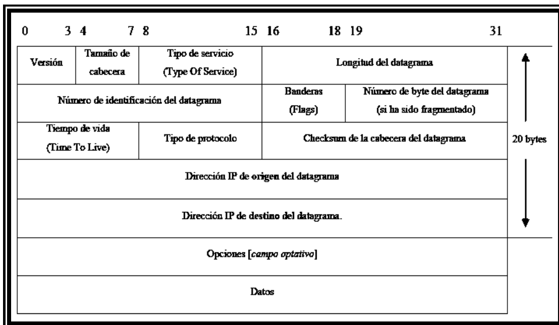
Figura 3.17.- Estructura de un datagrama IP v4.
