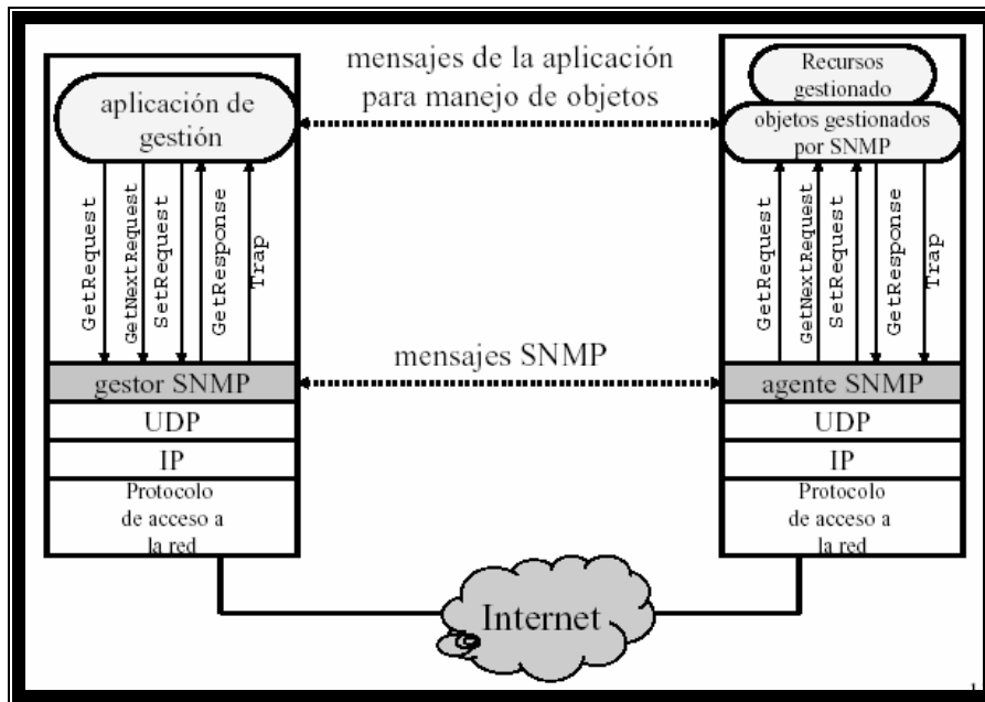
Figura 5. Elementos dentro de un entorno gestionado por SNMP .
