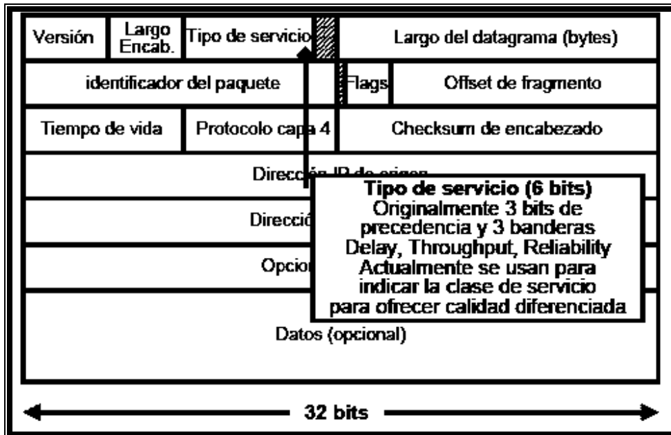
Figura 3.20.- Estructura de un datagrama IP v4, tipo de servicio.
