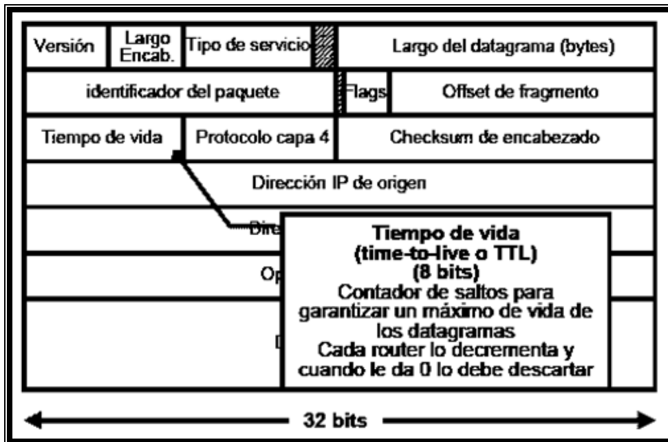
Figura 3.25.- Estructura de un datagrama IP v4, TTL.
