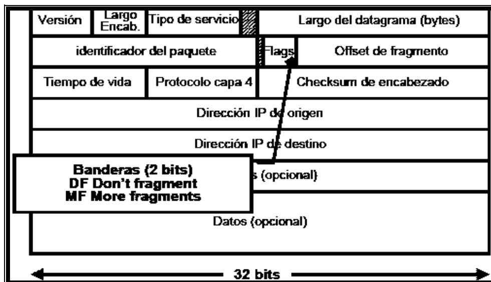
Figura 3.23.- Estructura de un datagrama IP v4, Banderas.
