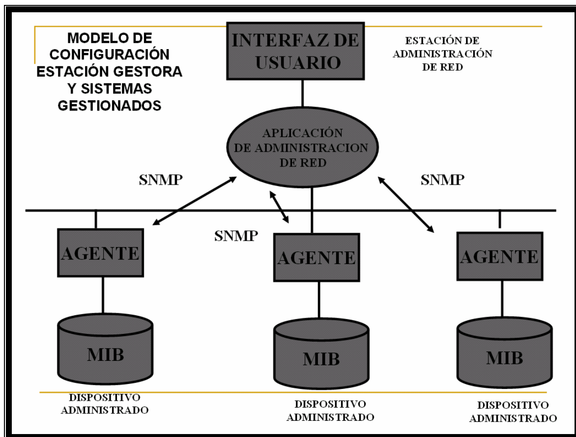
4.31.- Entorno de Gestión de SNMP y Monitorización en la Herramienta de Gestión.
