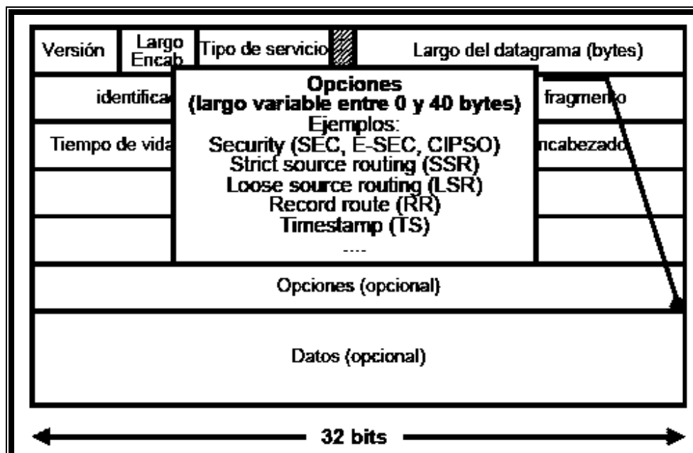
Figura 3.31.- Estructura de un datagrama IP v4, opciones.
