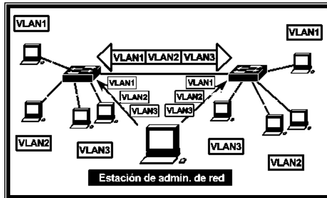
Figura 1.16.- VLAN estáticas
