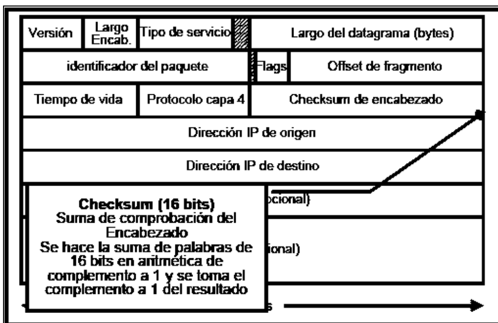
Figura 3.27.- Estructura de un datagrama IP v4, Checksum.
