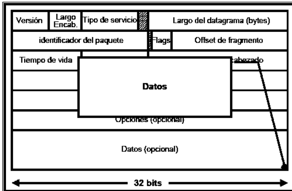
Figura 3.32.- Estructura de un datagrama IP v4, Datos.
