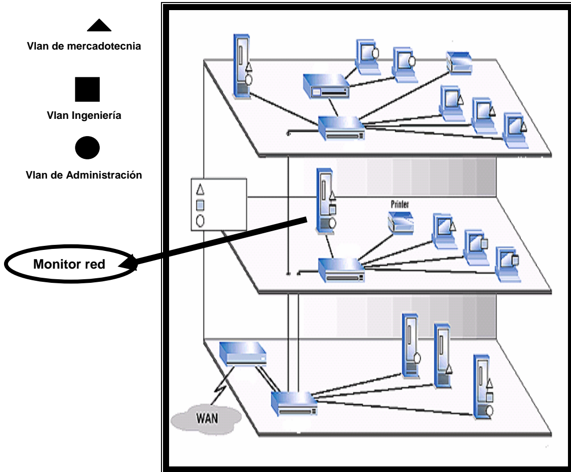
Figura 3.15. Monitoreo en una empresa con VLAN's
