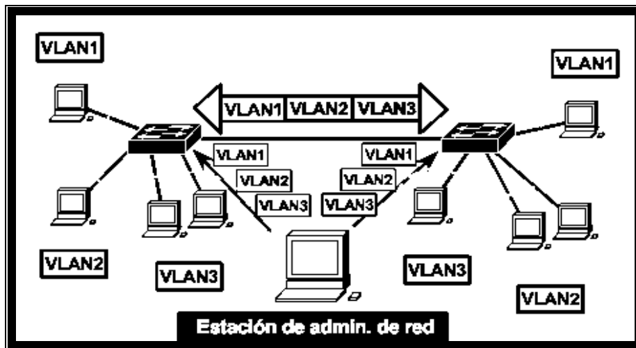
Figura 3.- VLAN estáticas
